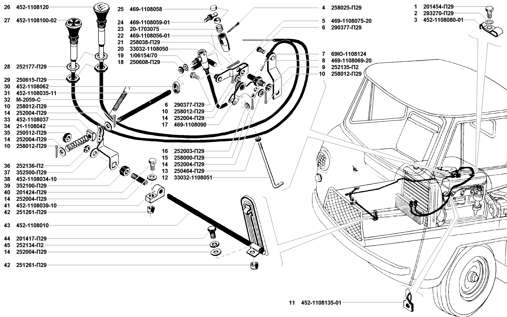
Рис. 27. Привод управления дроссельной и воздушной заслонками (1008) Fig. 27. Throttle and choke control (1108)
